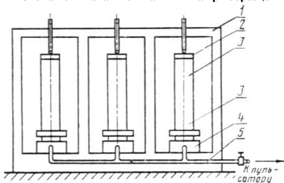
Схема испытательной машины на три образца
